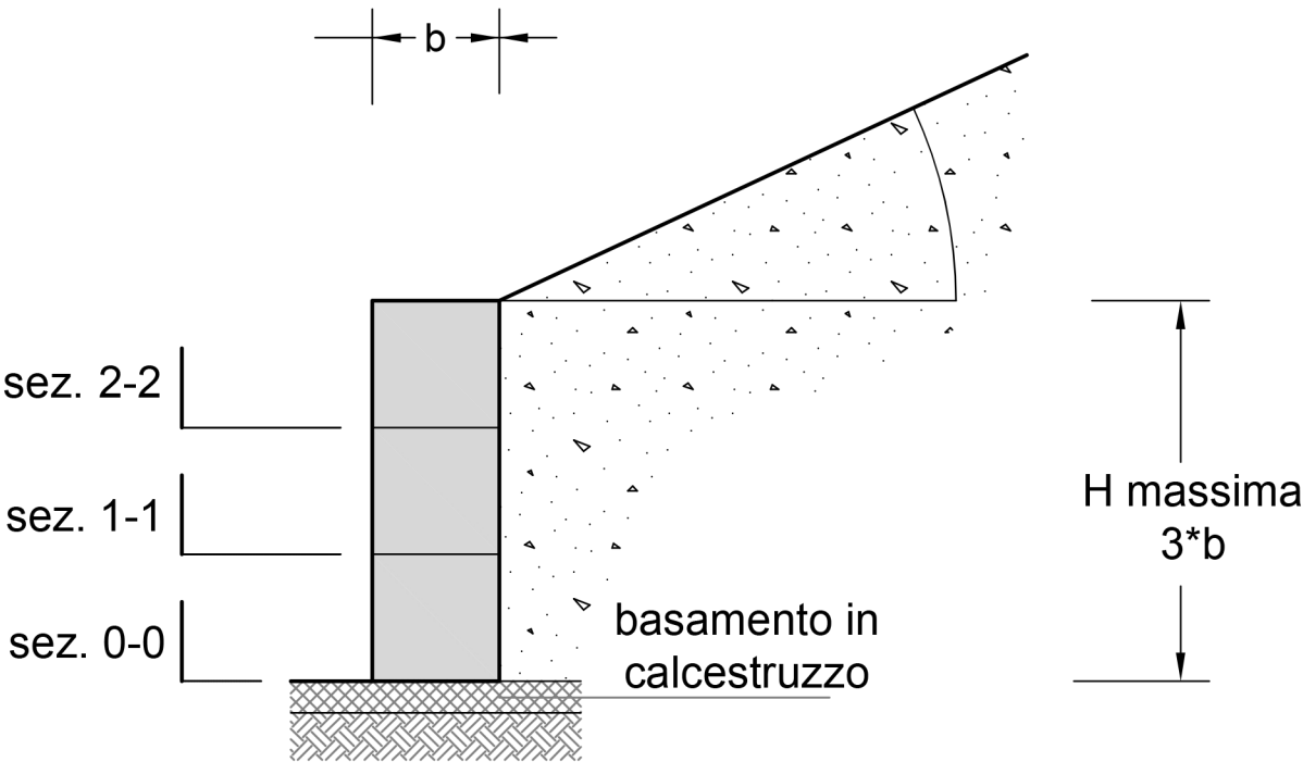
modalità di carico sezioni di verifica 3 blocchi
