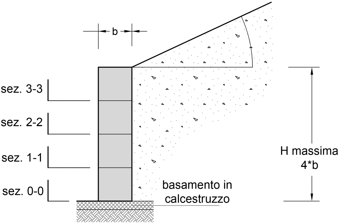
modalità di carico sezioni di verifica 4 blocchi
